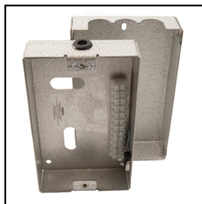
Montageboks m/klemmer DIM: B107xH167xD35
